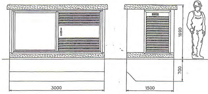
Pohľad na trafostanicu M 1:50
